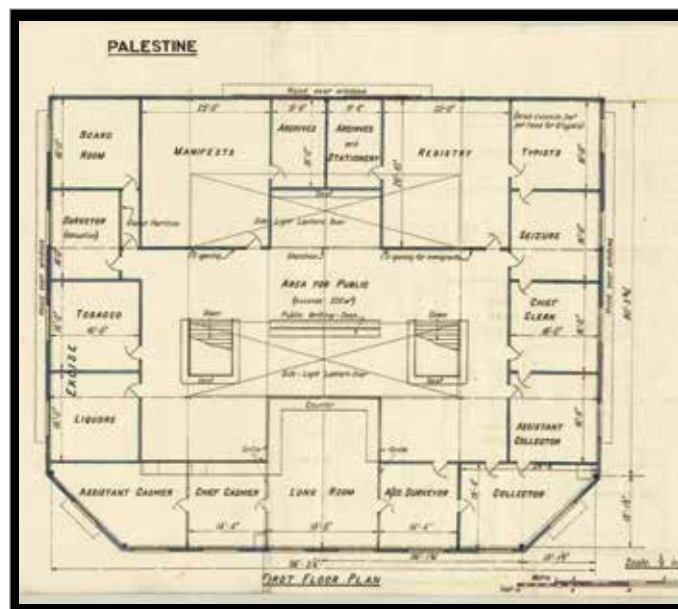
תוכנית בית המכס החדש, אפריל 1935: בתוכנית לא מופיעים משרדי הגירה ומשרד הבריאות. ארכיון המדינה
