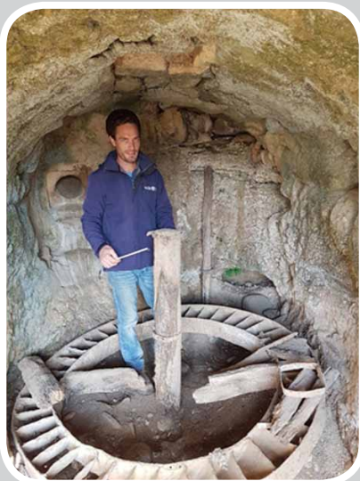
גלגל כפות וציר עץ כפי שנמצאו בחפירת הטחנה
