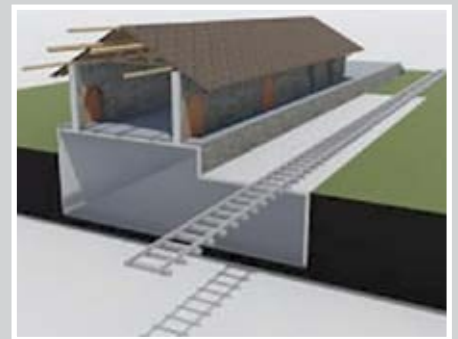
חלופה סכמטית של בנייה תת-קרקעית לבינוי החדש תחת בית המחסנים שישוחזר 'וכמן אדריכלים' ו'מעשה שימור'
